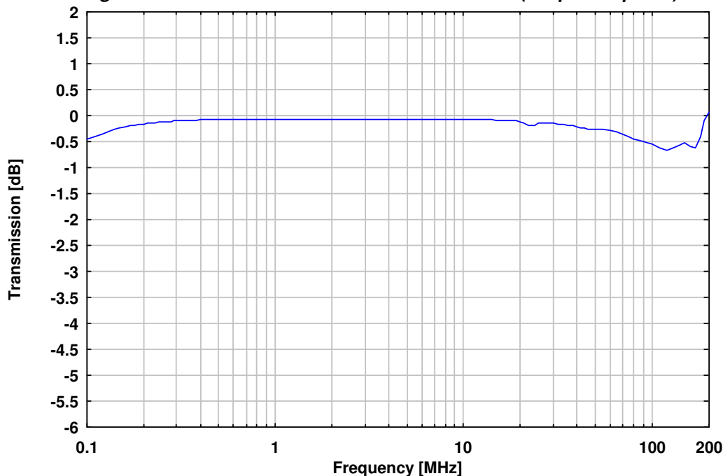
Spannungsteilungsmaß Prüflingsklemmen – N-Buchse (Spezialadapter erforderlich) Voltage division ratio EuT-Terminals to N-connector (adapter required)
