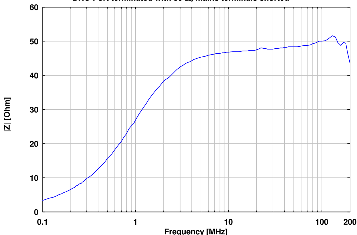
Impedanz an den Prüflingsklemmen (Kalibrieradapter KA 8125 erforderlich), BNC mit 50 \Omega Abschluss, Speiseklemmen kurzgeschlossen Impedance at EuT-Terminals (Calibration Adapter KA 8125 required), BNC-Port terminated with 50 \Omega , mains terminals shorted
